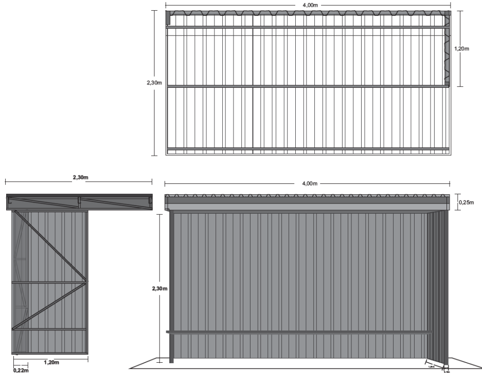
VISTA SUPERIOR DETALHES ESTRUTURA
